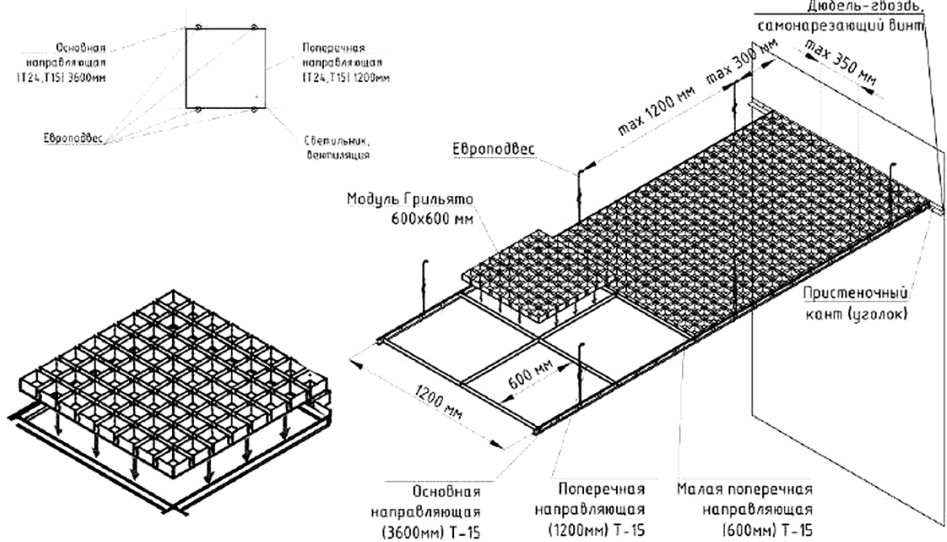
Расположение подвесов при монтаже светильников.
